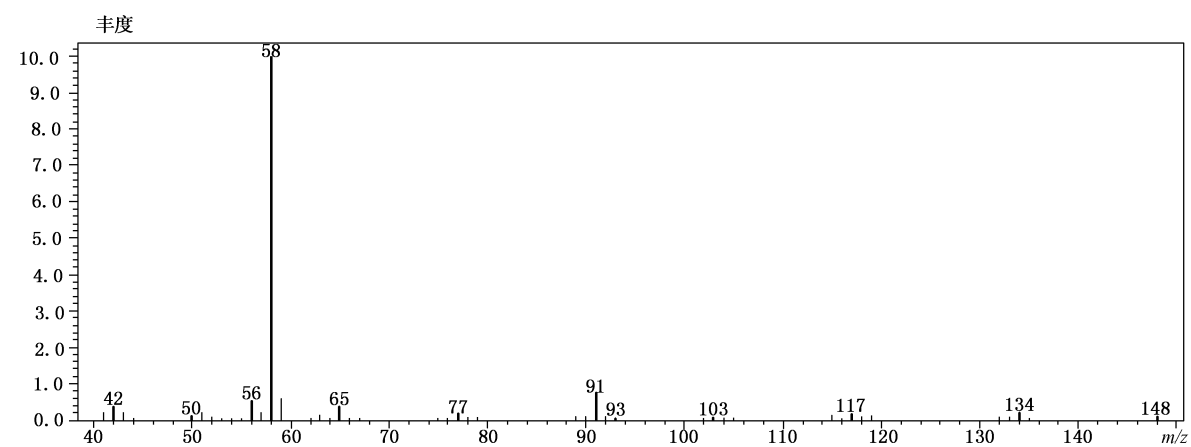
图 B.2 甲基苯丙胺质谱图
